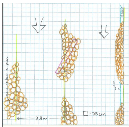
Figure 28. Plan détaillé du déflecteur P-035 du ruisseau des Pères
