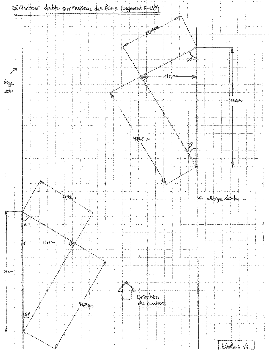
Figure 23. Plan technique du déflecteur double P-035 sur le ruisseau des Pères
