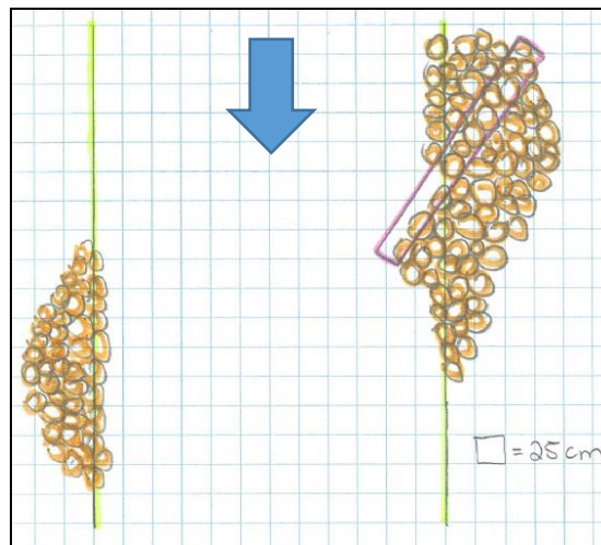
Figure 35. Plan détaillé du déflecteur M-005 du ruisseau Maltais
