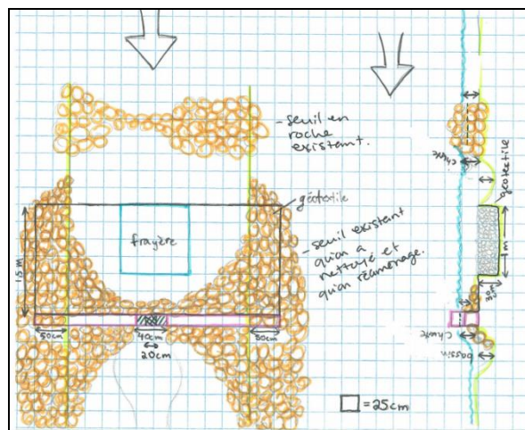
Figure 27. Plan détaillé du seuil P-036 du ruisseau des Pères
