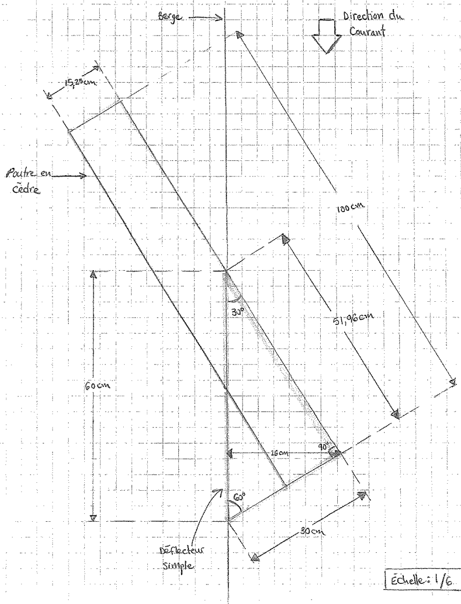
Figure 21. Plan technique des déflecteurs simples (segments M-005 et M-018) sur le ruisseau Maltais
