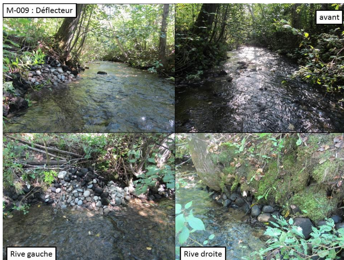
Figure 8. Aménagement du déflecteur M-009
