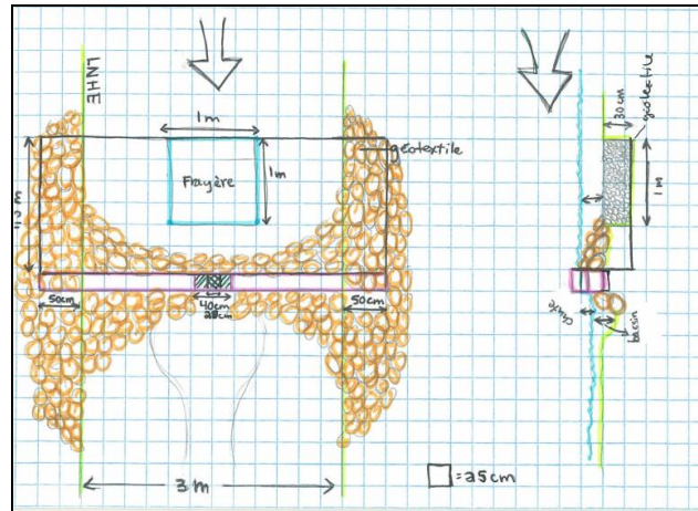
Figure 30. Plan détaillé du seuil P-032 du ruisseau des Pères
