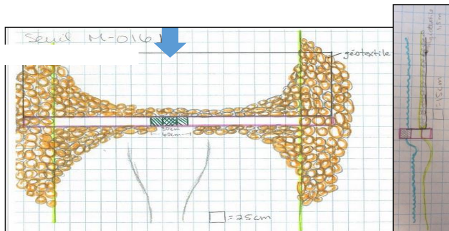
Figure 32. Plan détaillé du seuil M-016 du ruisseau Maltais
