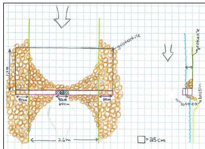
Figure 25. Plan détaillé du seuil P-040 du ruisseau des Pères
