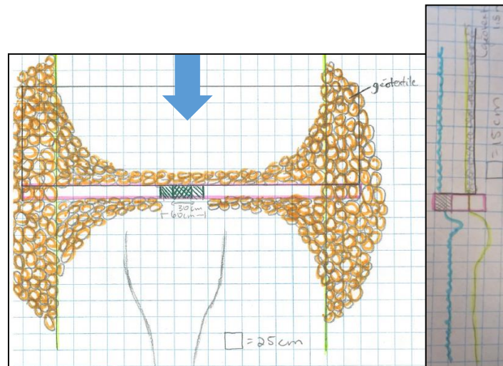
Figure 31. Plan détaillé du seuil M-020 du ruisseau Maltais
