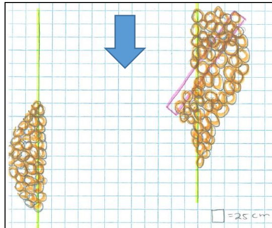
Figure 33. Plan détaillé du déflecteur M-016 du ruisseau Maltais
