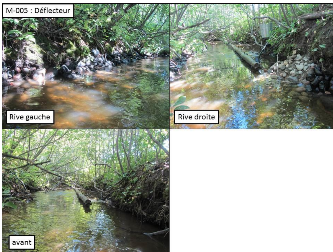
Figure 9. Aménagement du déflecteur M-005
