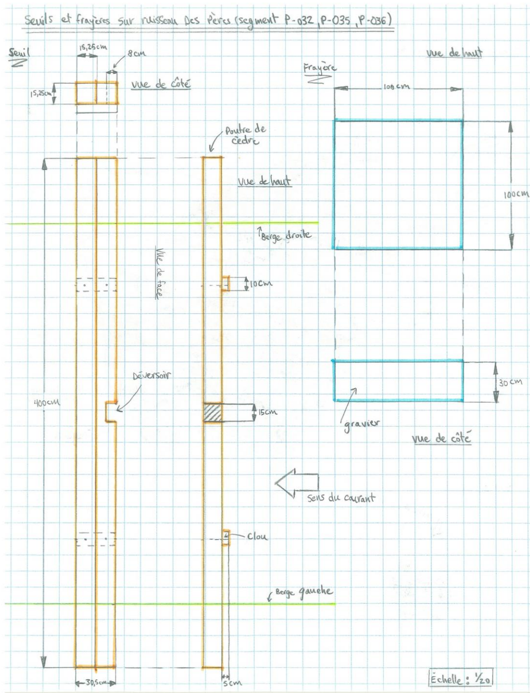
Figure 22. Plan technique des seuils et frayères sur le ruisseau des Pères (segments P-032, P-035, P-036)
