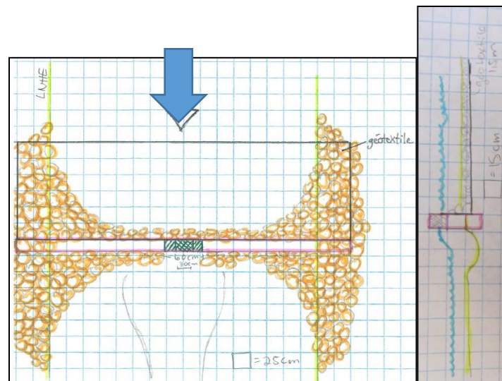
Figure 34. Plan détaillé du seuil M-013 du ruisseau Maltais
