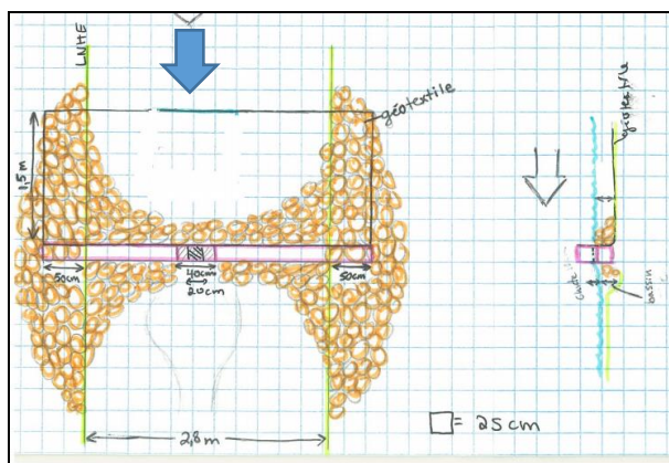
Figure 29. Plan détaillé du seuil P-035 du ruisseau des Pères
