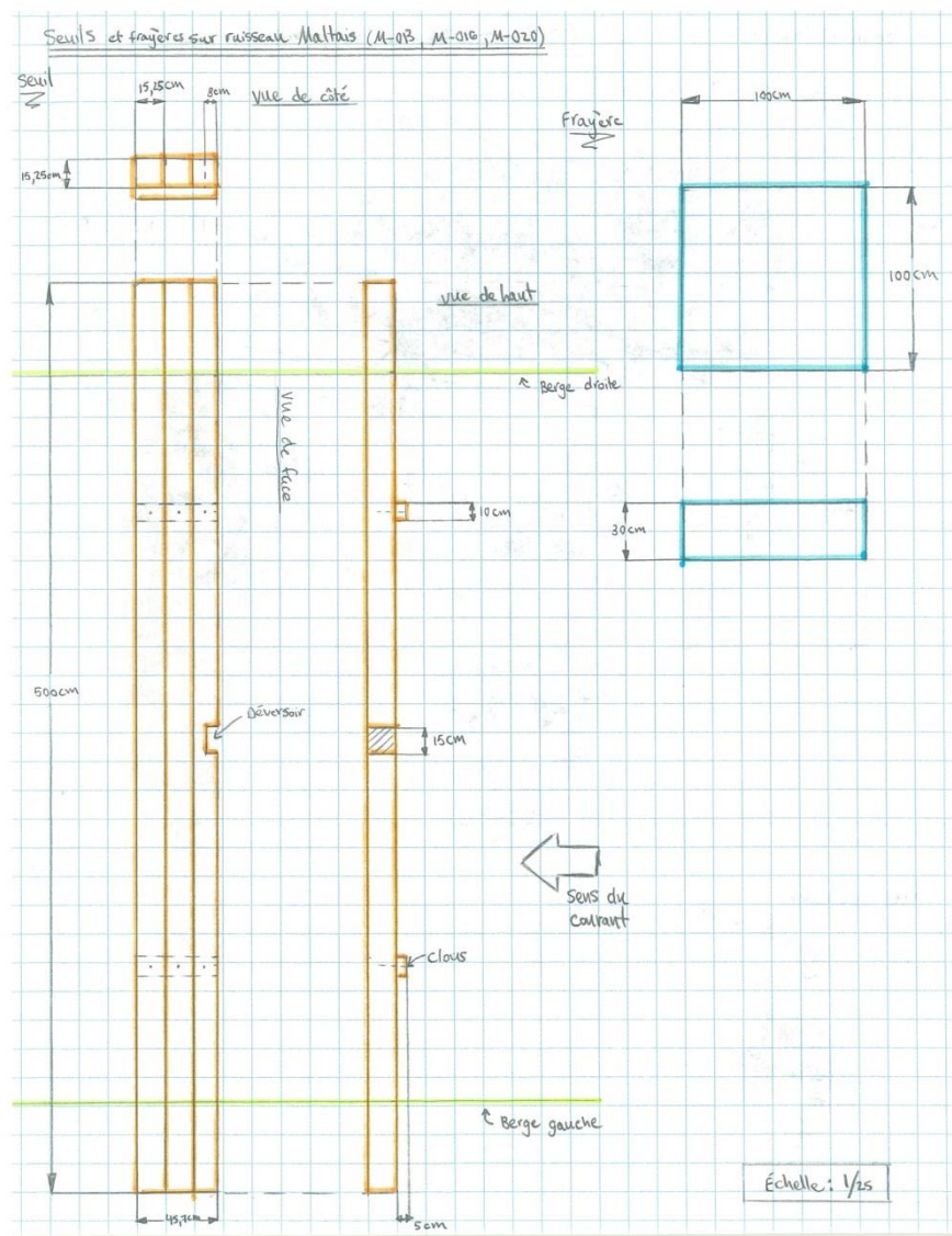
Figure 20. Plan technique des seuils sur le ruisseau Maltais (segments M-013, M-016, M-020)
