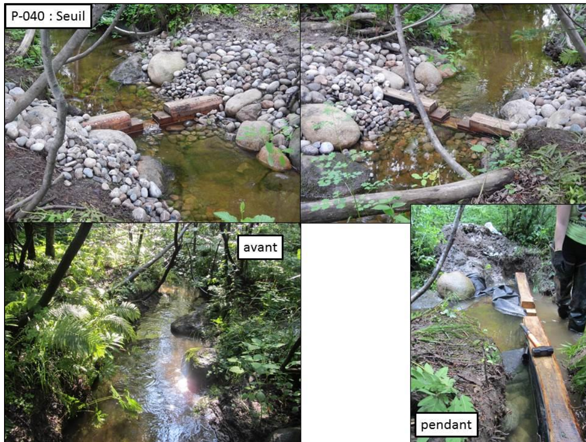
Figure 11. Aménagement du seuil P-040
